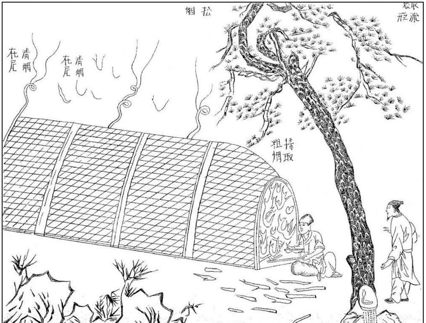
Pl. VII. Préparation du noir de fumée destiné à la fabrication de l'encre de Chine au moyen de bois résineux.
