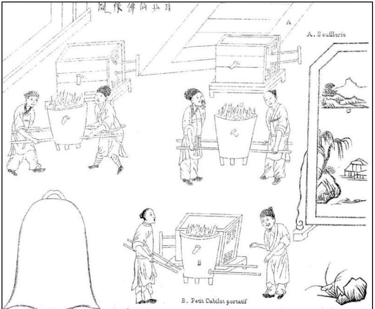
Pl. V. Fonte des cloches et des statuettes de Bouddha.
