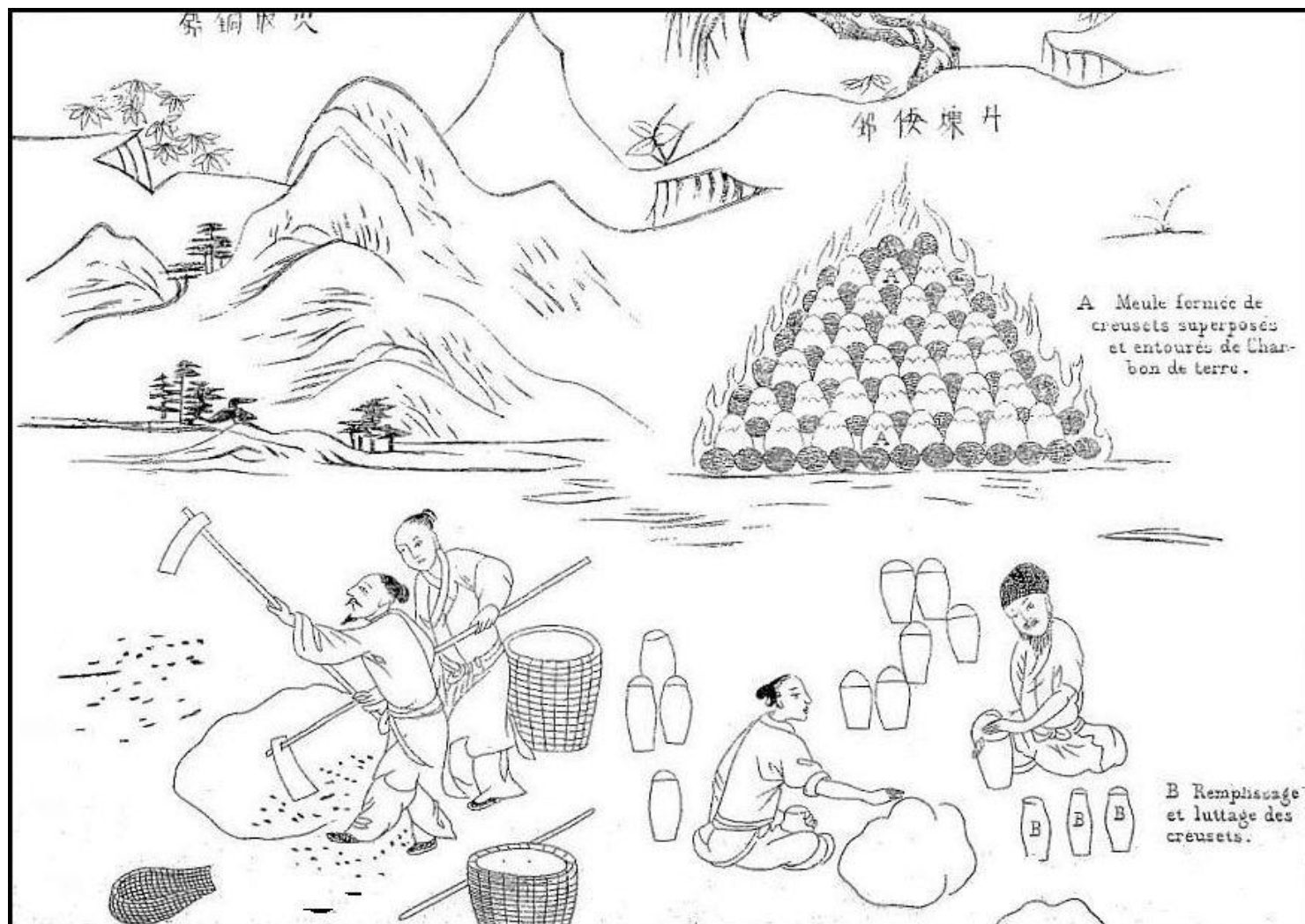
Pl. II. — Extraction du zinc (plomb japonais).
